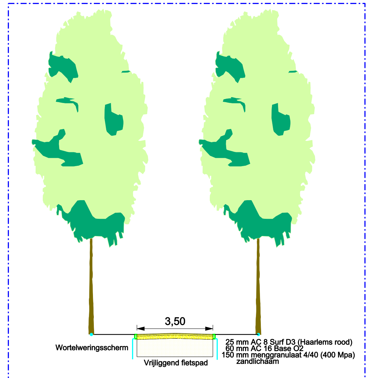
Doorsnede A-A
