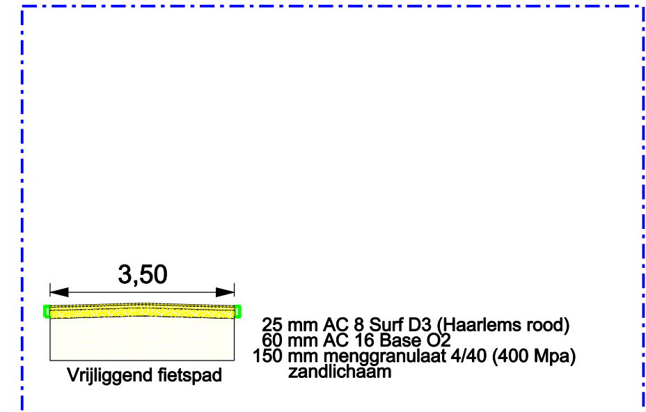
Doorsnede B-B
